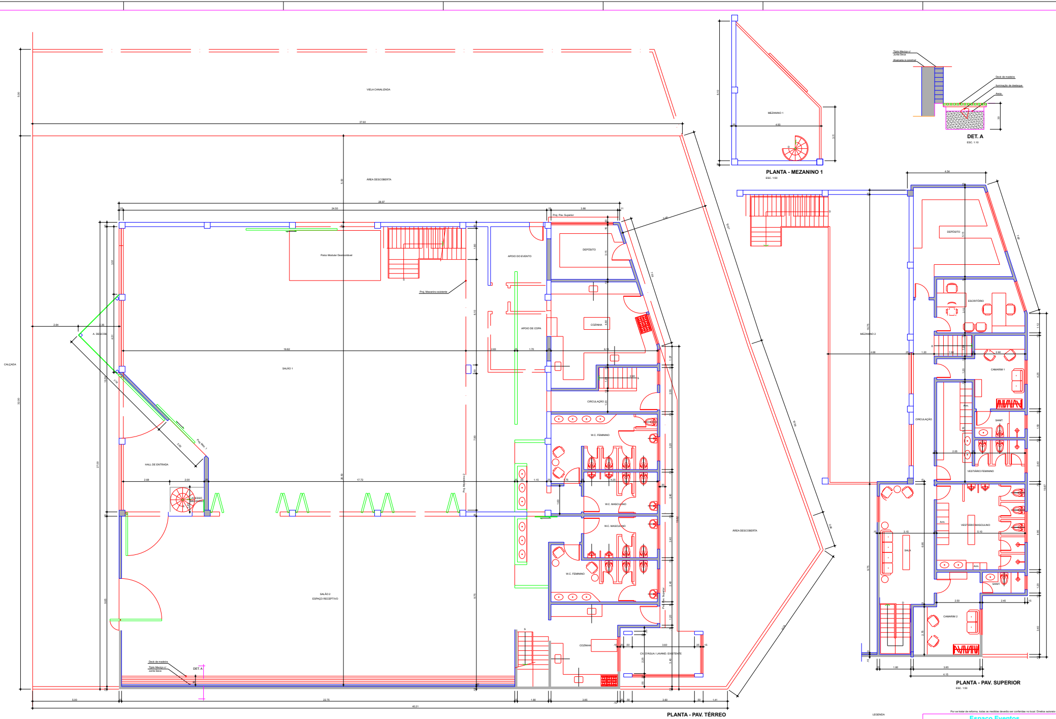
PLANTA - PAV. TÉRREO ESC. 1:50
